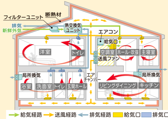
【Airフローシステムの空気の流れ】
