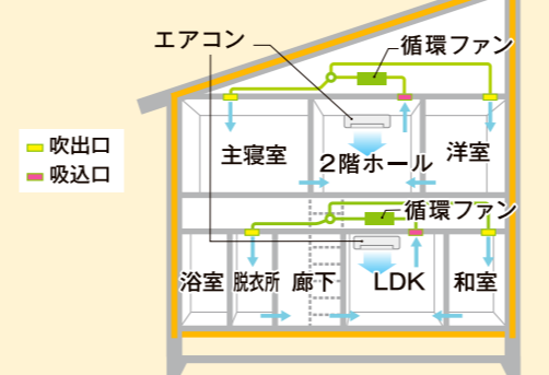
【Airフローシステムの空気の流れ】
