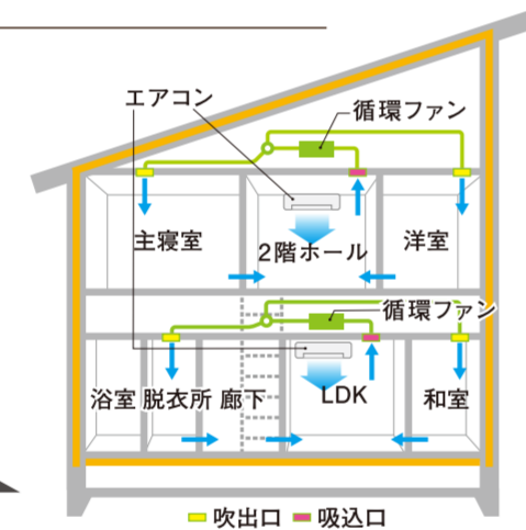
Airフローシステム 空気の流れ
